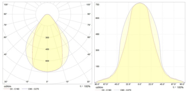
Courbes photométriques
