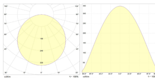
Courbes photométriques
