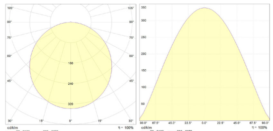
Courbes photométriques
