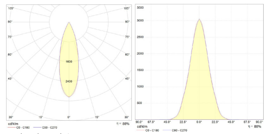
Courbes photométriques
