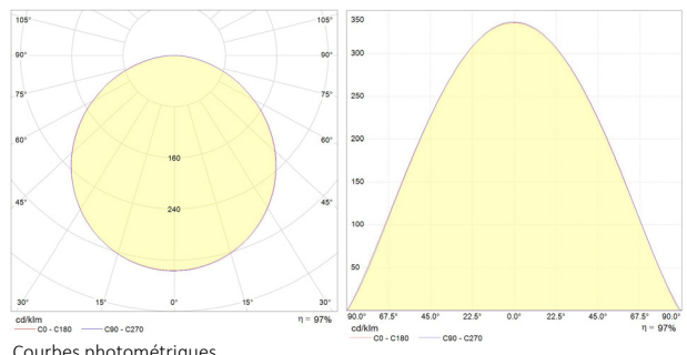
Courbes photométriques
